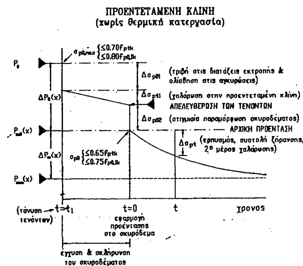
Σχήμα Σ 4.1α Απώλειες προέντασης σε δεδομένη διατομή (προένταση πριν από την έγχυση του σκυροδέματος)
