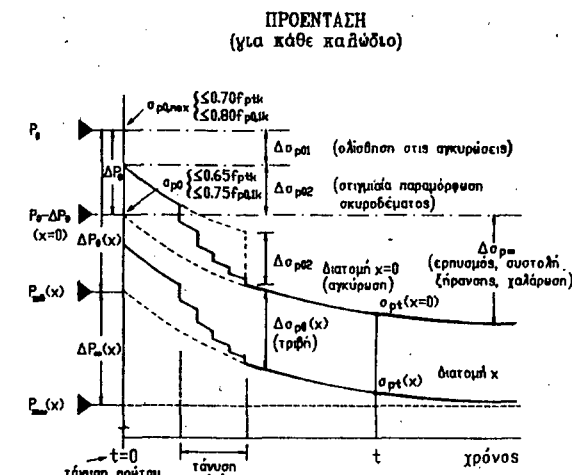
Σχήμα Σ 4.1β Απώλειες προέντασης σε δεδομένη διατομή (προένταση μετά από την σκλήρυνση του σκυροδέματος)
